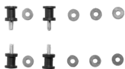
Anschraubbare Auflagepunkte (M5, M6) zur Befestigung des Gepäckträgers
